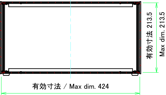
C-C ( 1 : 6 )
