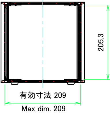
A-A ( 1 : 6 )
